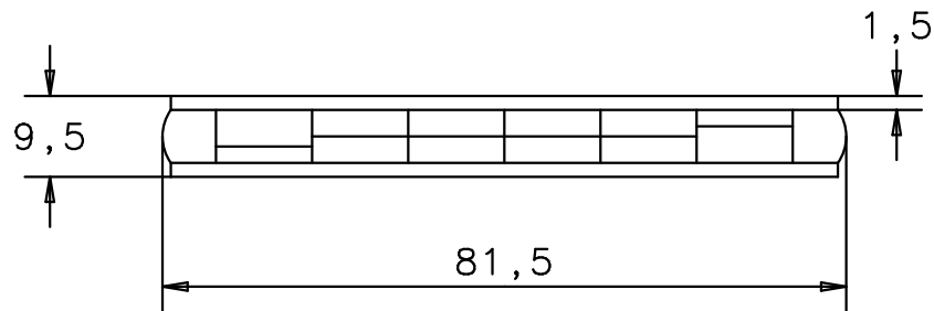
Draufsicht top view
