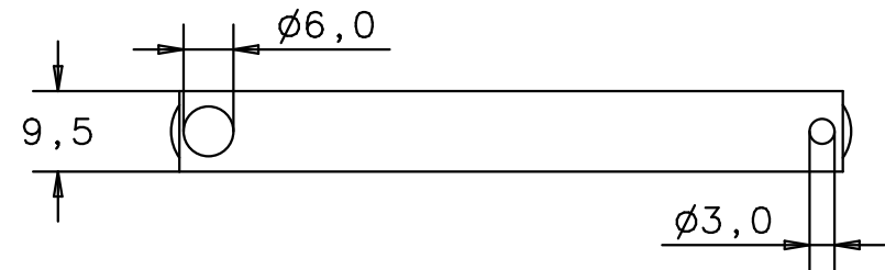
Unteransicht bottom view
