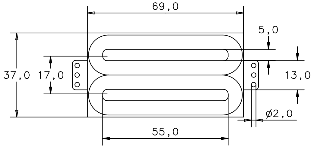
Draufsicht top view
