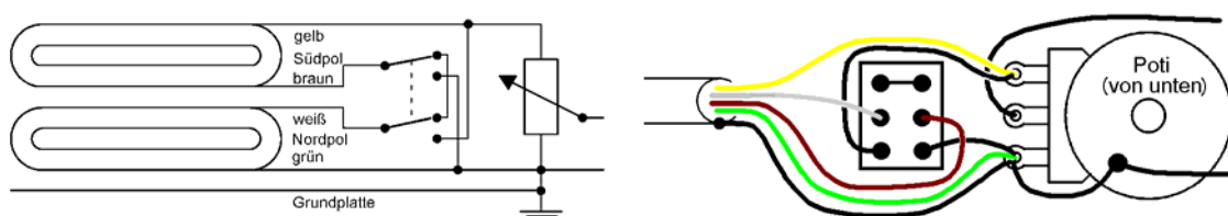
Umschaltung parallel / seriell mit zweipoligem Umschalter
