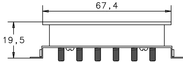
Vorderansicht front view
