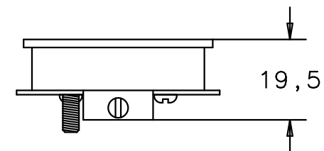
Seitenansicht von rechts side view right
