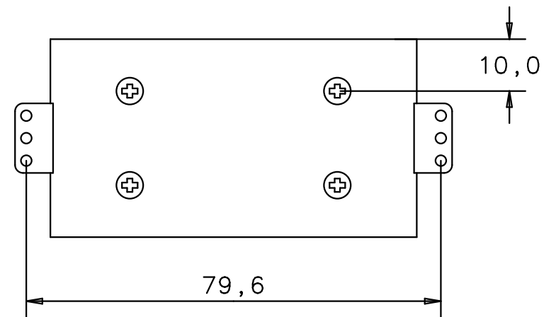
Seitenansicht von rechts side view right
