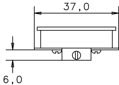
Seitenansicht von links side view left
