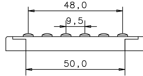
Rückansicht back view
