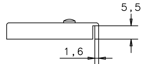
Seitenansicht von rechts side view right
