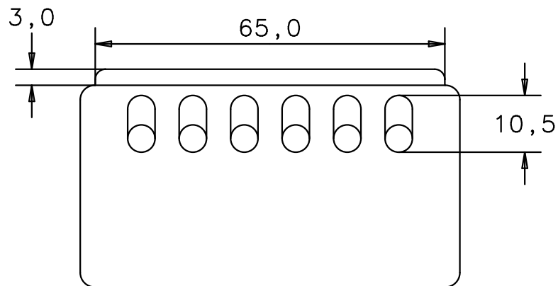
Draufsicht top view
